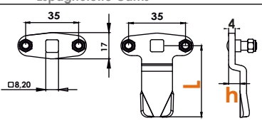
Espagnolette Cams
