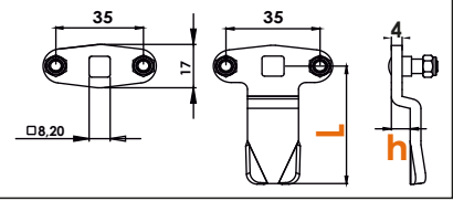
Espagnolette Cams
