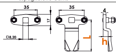
Espagnolette Cams
